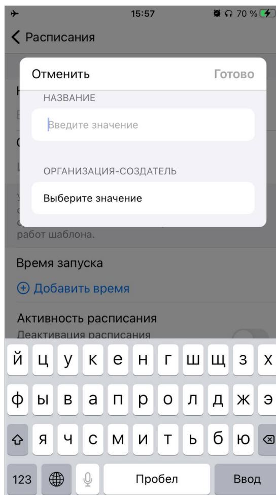
Рис. 2.106: Создание расписания
