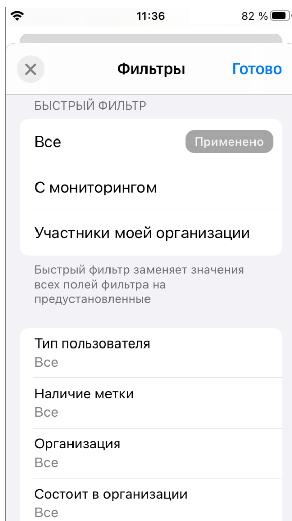
Рис. 2.99: Фильтр пользователей
