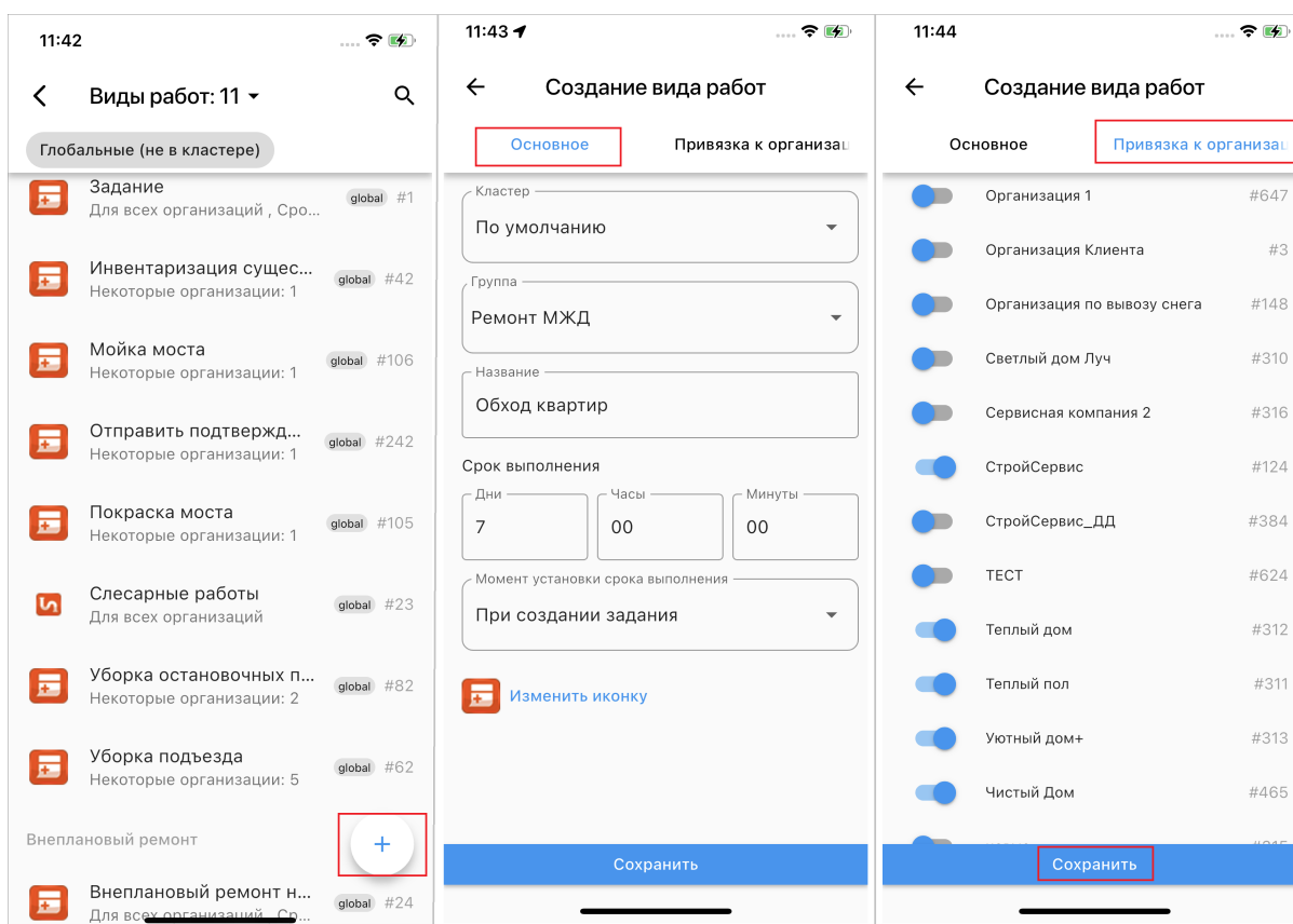
Рис. 2.111: Создание вида работ
