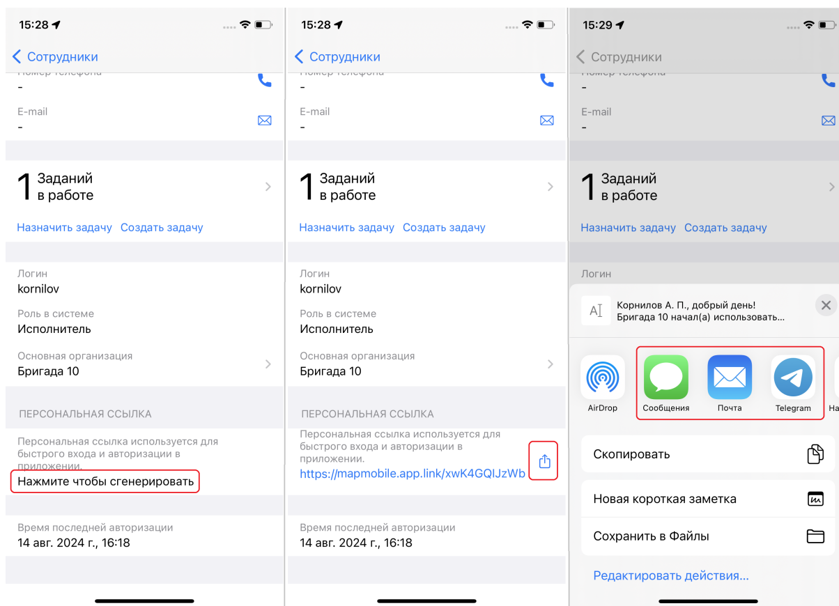
Рис. 2.103: Формирование и отправка ссылки для нового пользователя
