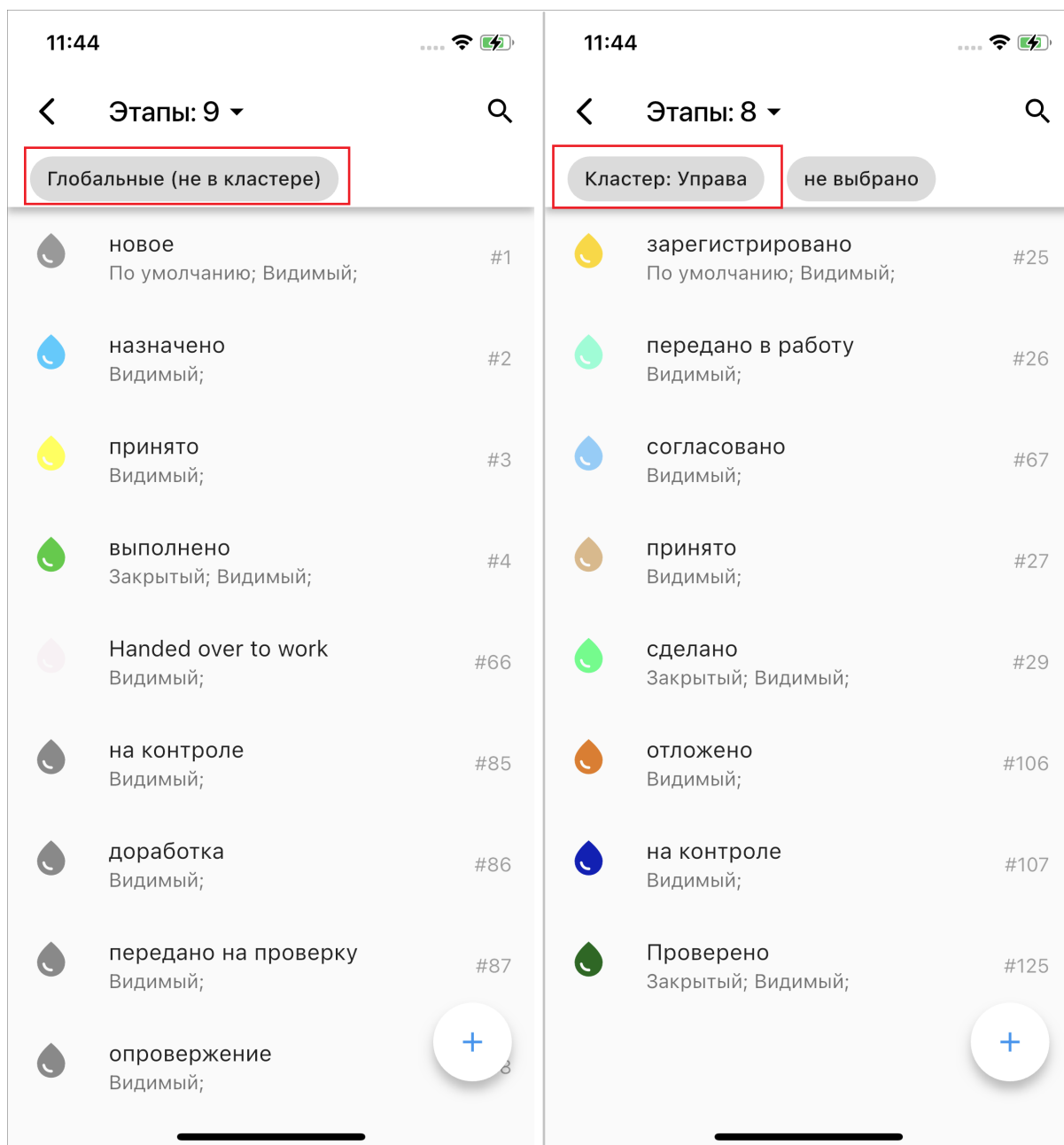
Рис. 2.112: Фильтр кластеров
