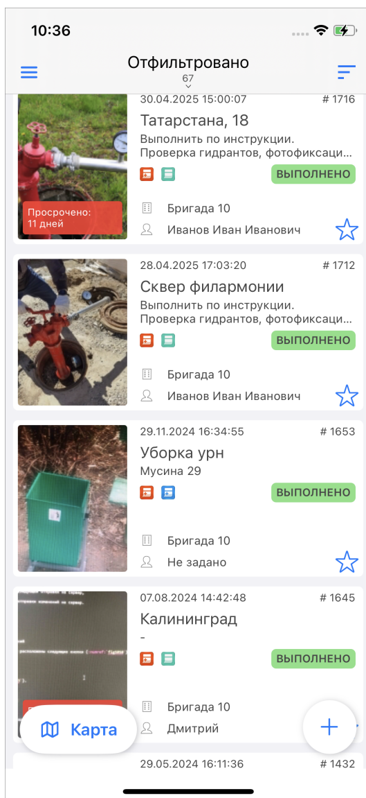
Рис. 2.26: Отфильтрованные задания
