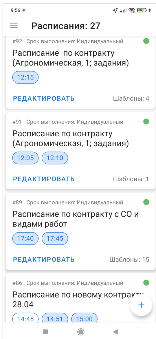
Рис. 2.105: Список расписаний
