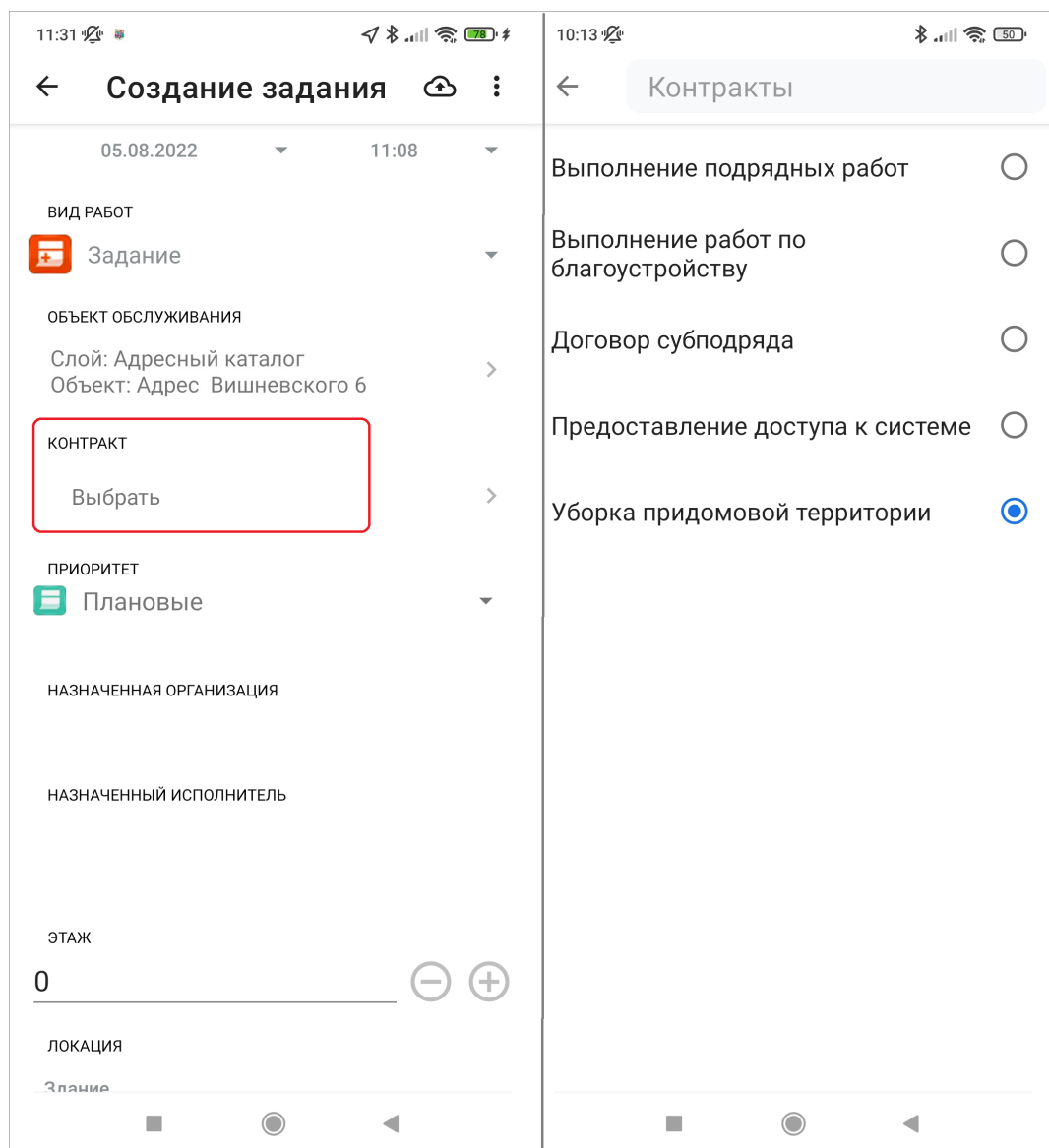
Рис. 2.48: Прикрепление контракта
