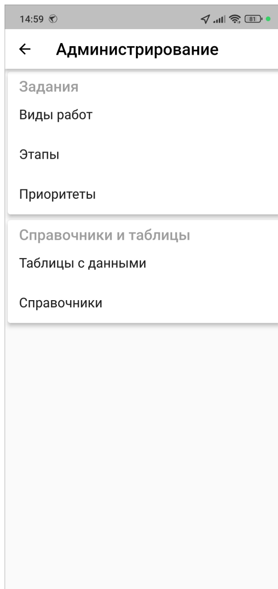
Рис. 2.106: Раздел «Администрирование»
