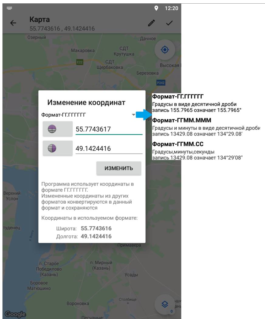
Рис. 2.51: Изменение координат
