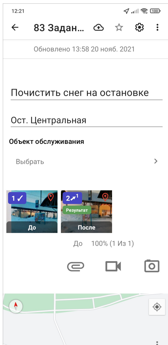
Рис. 2.60: Отображение «Фото-связей»
