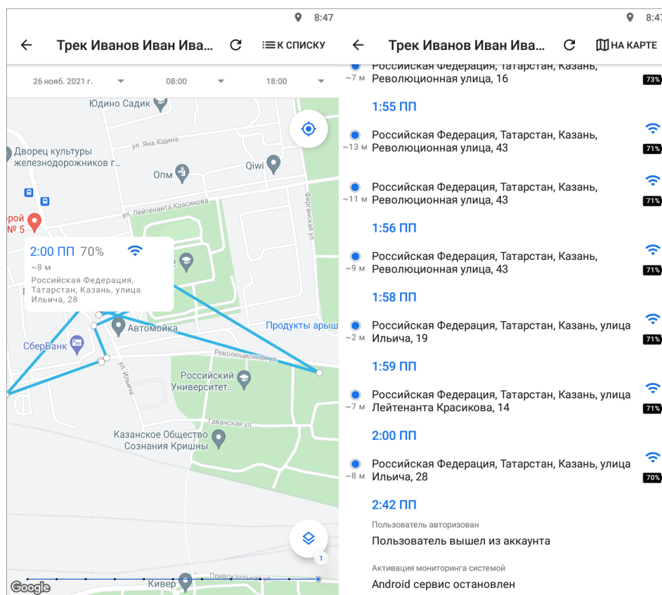
Рис. 2.63: Просмотр трека
