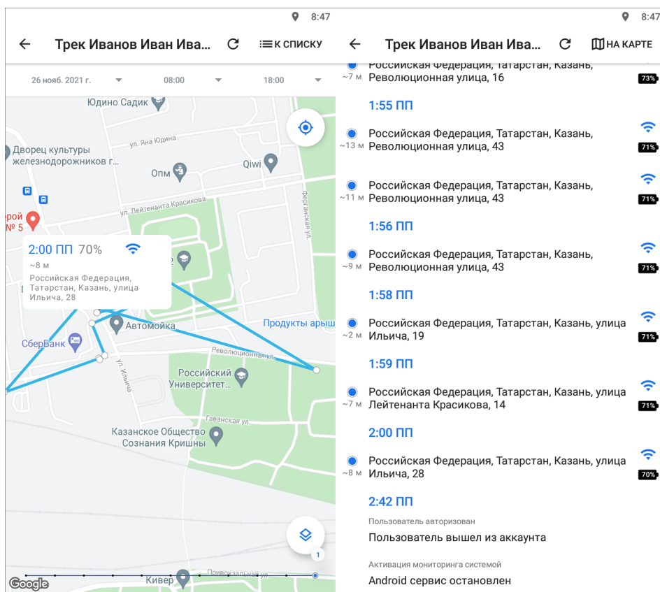
Рис. 2.98: Просмотр трека
