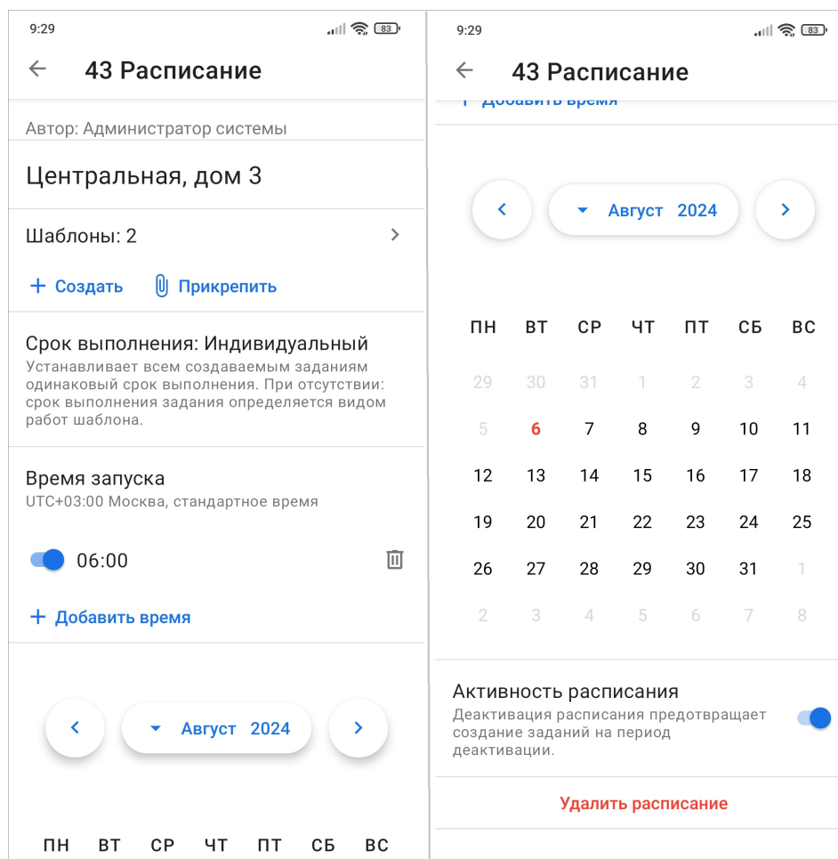
Рис. 2.104: Создание расписания
