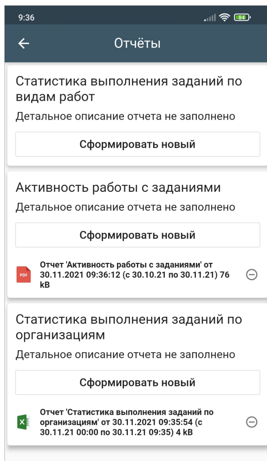
Рис. 2.117: Окно «Отчеты»
