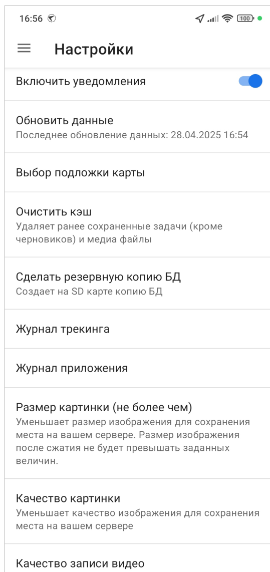
Рис. 4.1: Окно «Настройки»
