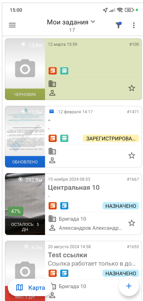
Рис. 2.29: Мои задания
