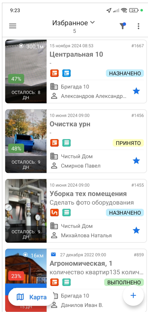
Рис. 2.21: Избранные задания
