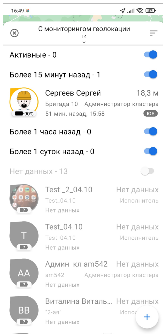
Рис. 2.96: Окно «Сотрудники»
