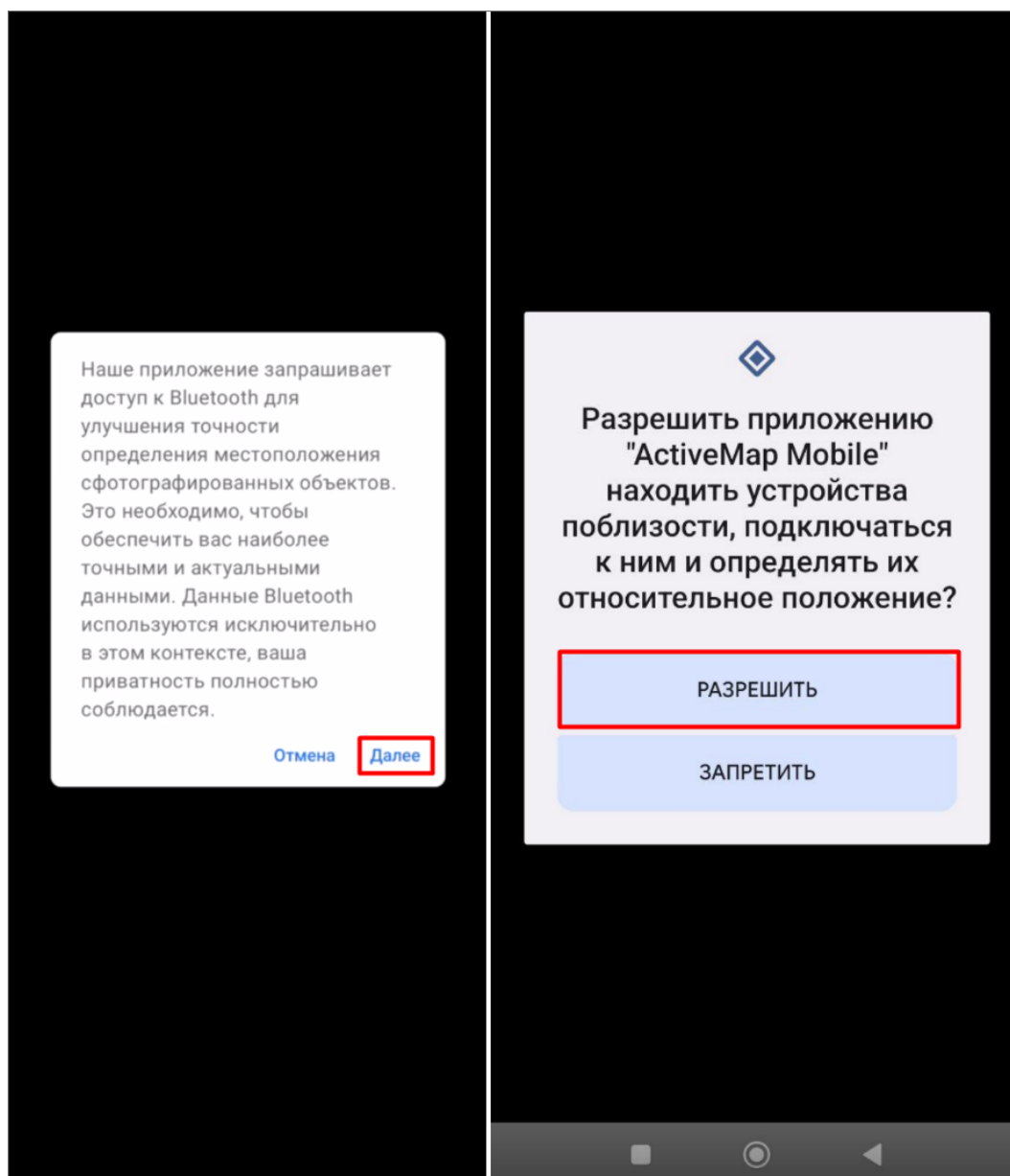
Рис. 2.119: Предоставление разрешений
