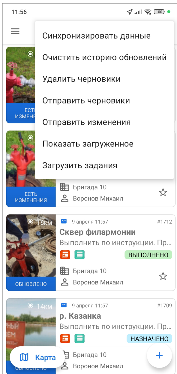
Рис. 2.24: Меню окна
