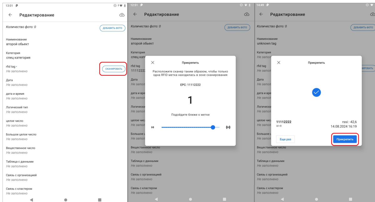
Рис. 2.121: Сканирование RFID-метки
