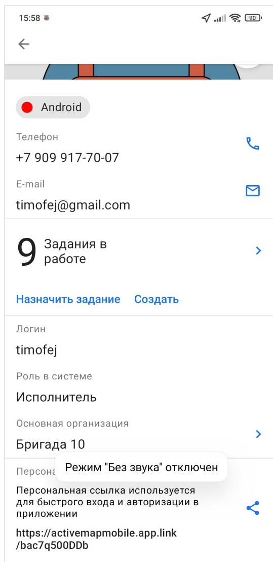
Рис. 2.64: Профиль сотрудника
