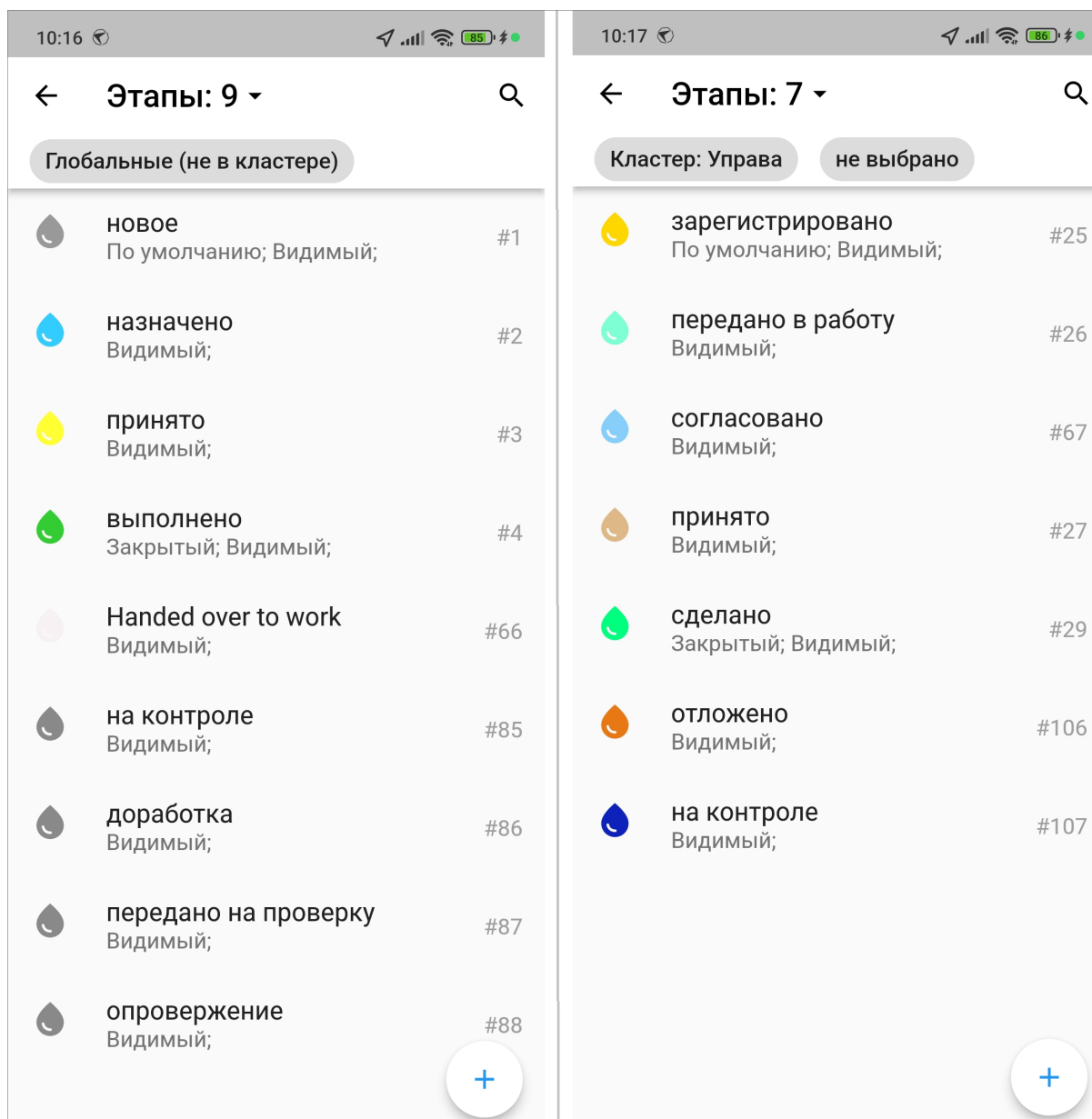
Рис. 2.108: Фильтр кластеров
